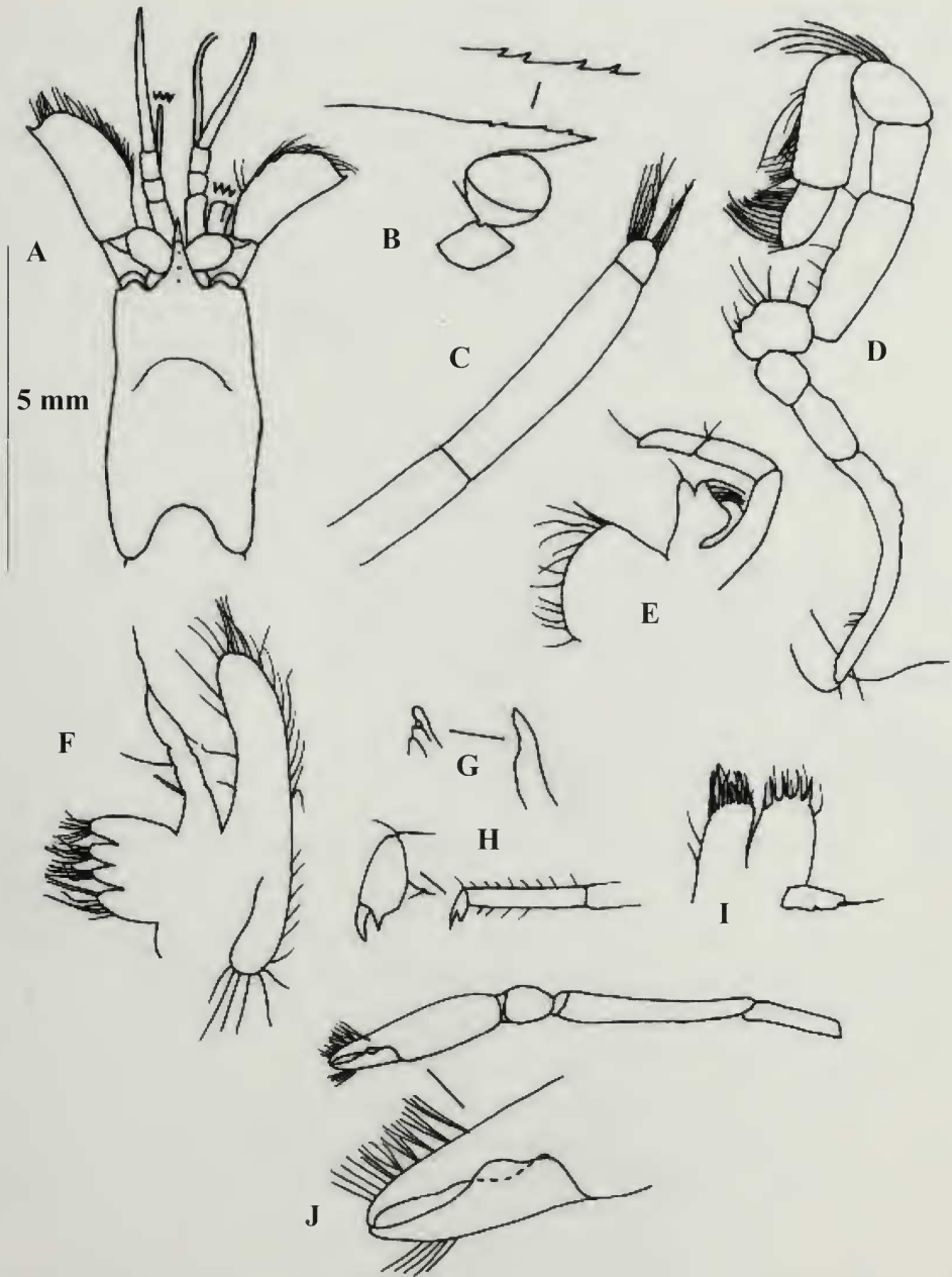
Figura 1. Spongiocaris goyi , especie nueva, A, vista dorsal del cefalotórax, B, vista lateral del rostrum, C, parte distal del maxilípodo 3, D, maxilípodo 2, E, maxilípodo 1, F, maxila, G, parte distal de la mandíbula, H, pereiópodo 2, I, maxilula, J, pereiópodo 3.
